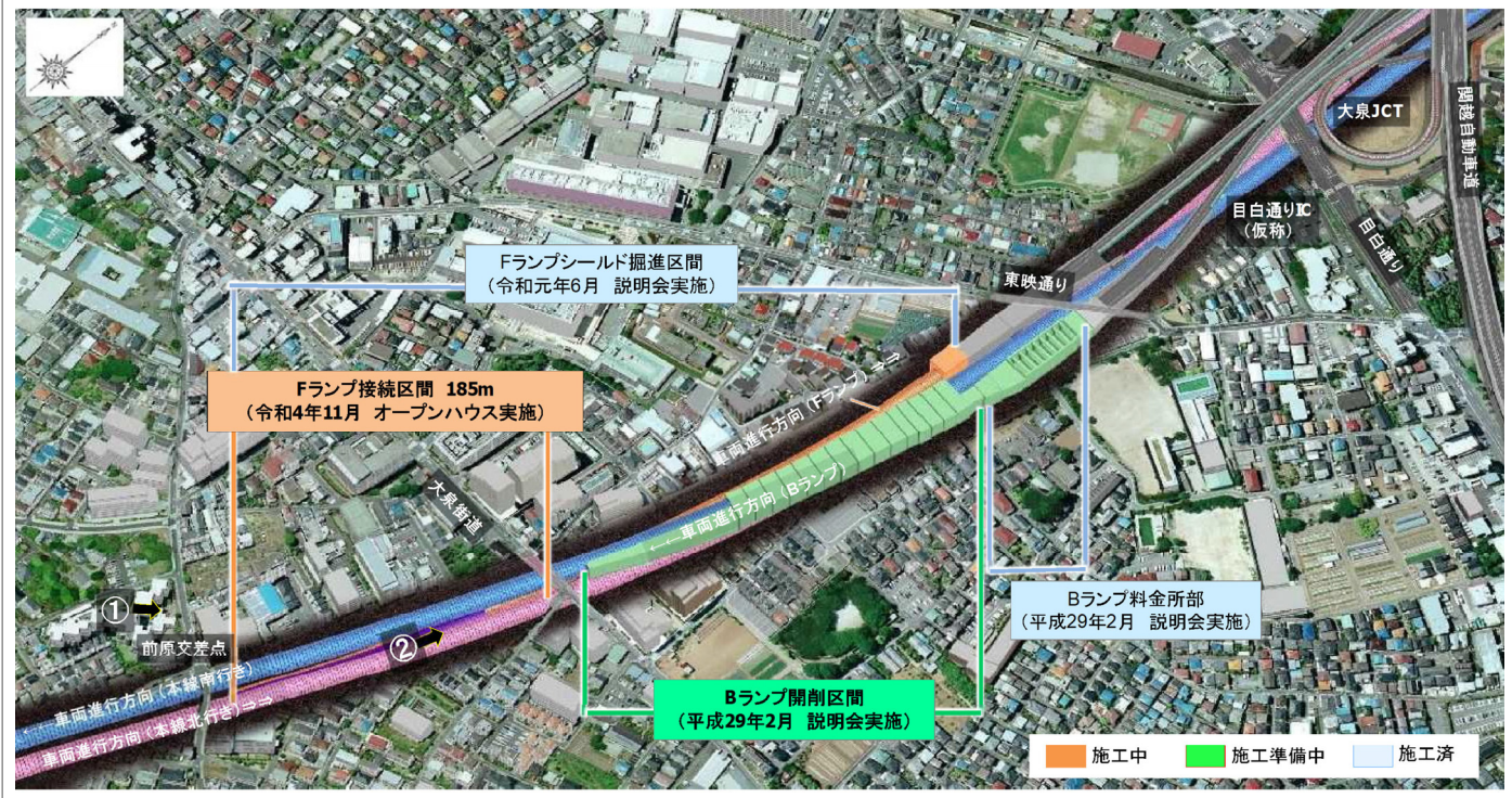
【工事概要図】
